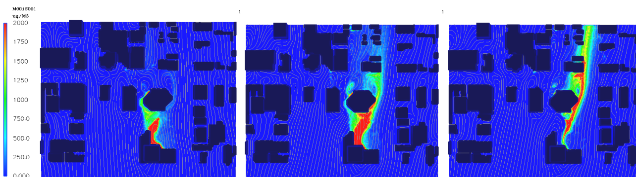
Figure 23 : lignes de courant et concentration en SF6 à 4h10, 4h20 et 4h30
