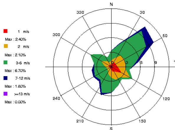
Figure 13 : rose des vents calculée à partir des échéances sans pluie
