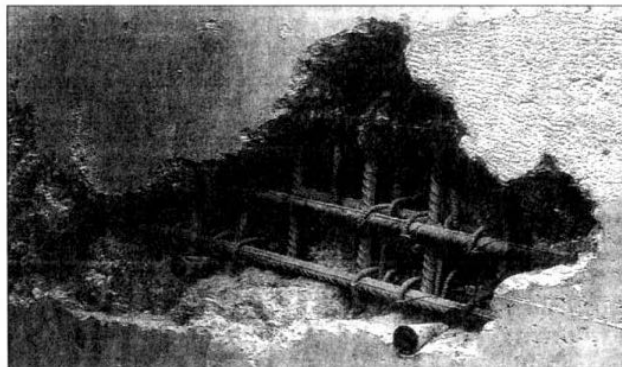
Photo d'un mur de la piscine du bâtiment où sera entreposé le combustible irradié de Flamanville. Ce cliché, comme beaucoup d'autres, a été pris en avril, après le décoffrage du béton. La ferraille à l'air, les enceintes du futur réacteur sont pleines de trous béants...
