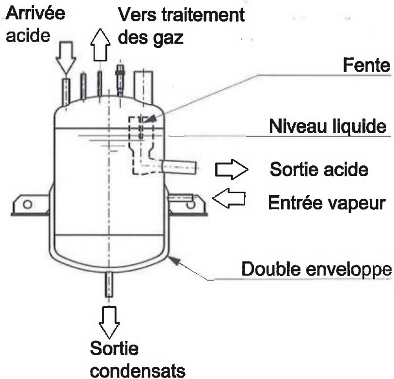
Figure 1 - Schéma descriptif du pot de passage 2220A-4017 de l'atelier T1
