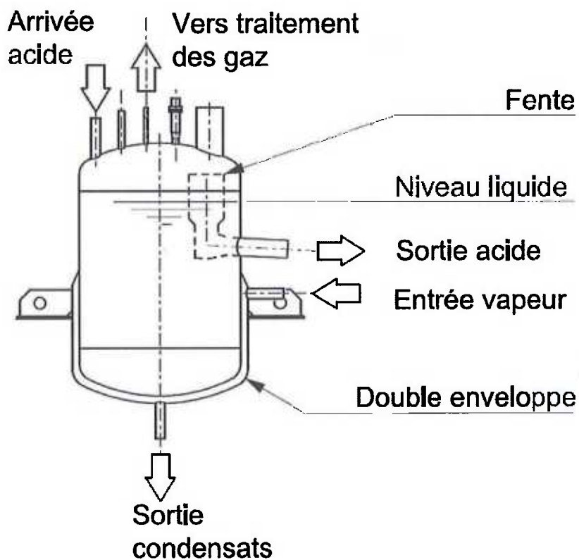
Figure 1 – Schéma descriptif du pot de passage 2220B-4017 de l'atelier R1
