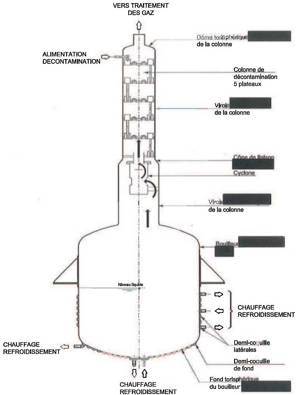
Figure 1 - Schéma descriptif de l'évaporateur R2 4120-21.
